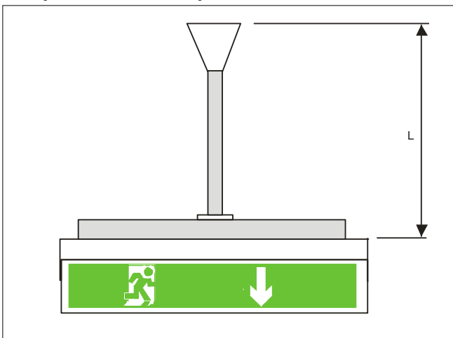
Suspension de tube pendentif
