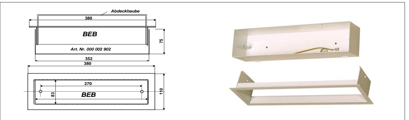
Flache Abdeckhaube
