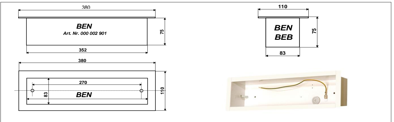
BEB-2 - Einbetonier-Gehäuse - 2-teilig
