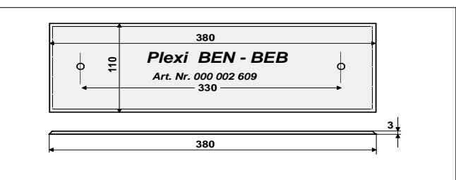
Flache Abdeckhaube
